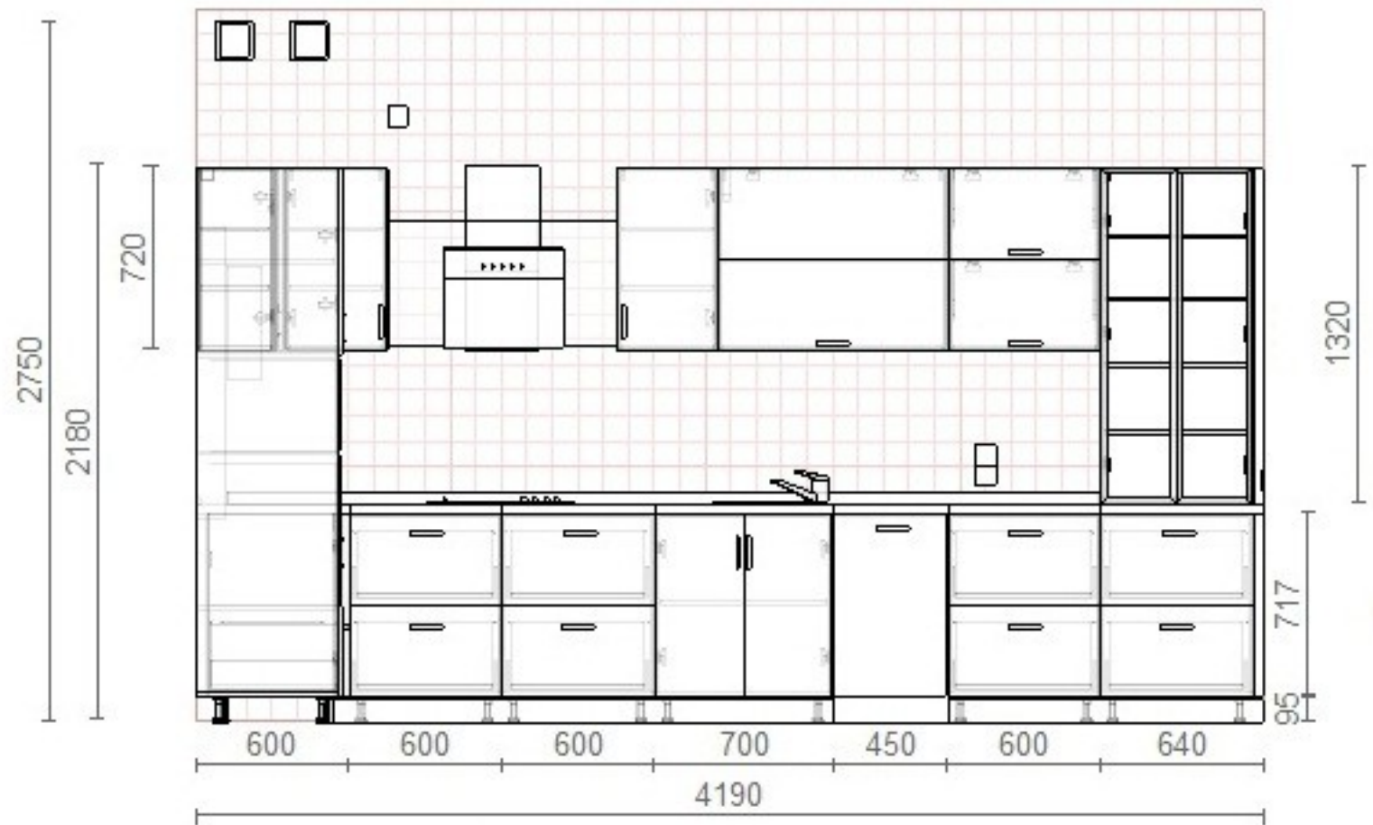
Фронтальный вид
